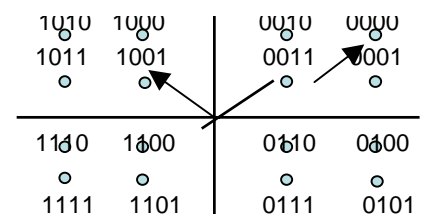
Konstellationsdiagramm bei 16-QAM Modulation
